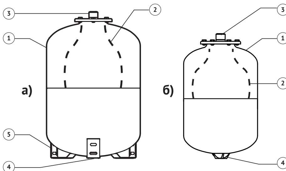
Рисунок 1 – Устройство расширительного бака а) – вертикальный; б) – подвесной
